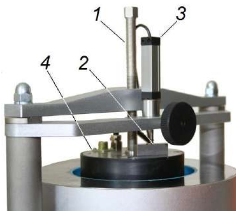
1 – винт нагружения; 2 – меры длины концевая плоскопараллельная (КМД); 3 – датчик перемещения; 4 – верхняя термоплита
