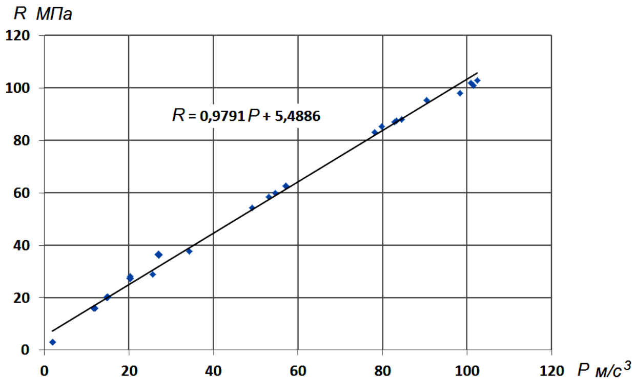
Рисунок 1 – Построение линейной градуировочной зависимости между параметром P и прочностью бетона R
