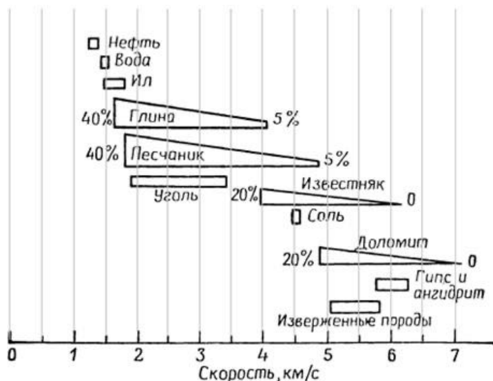
Рисунок 14 – Скорость продольных волн в породах различных типов. Для глин, песчаников, известняков и доломитов указана так же зависимость от пористости в процентах
