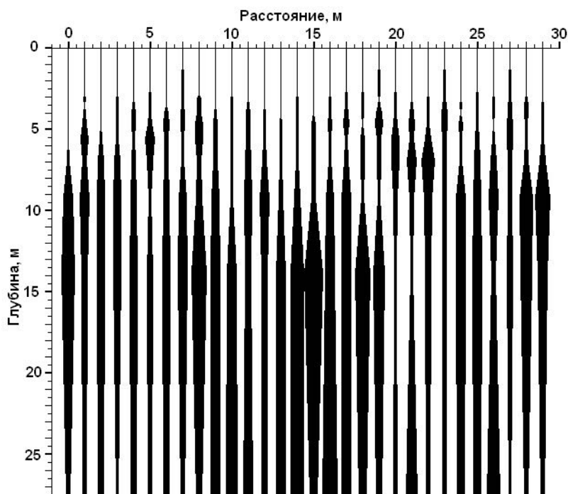
Рисунок 13 – Спектральный сейсмопрофиль грунта
