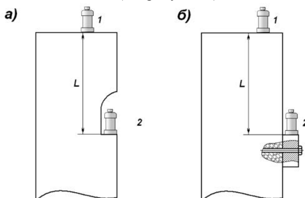
Рисунок 6 - Расположение сейсмоприемников на железобетонной свае
