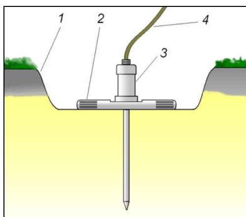
1 – верхний слой грунта; 2 – приспособление для крепления сейсмоприемника на грунт; 3 – сейсмоприемник; 4 – кабель сейсмоприемника
