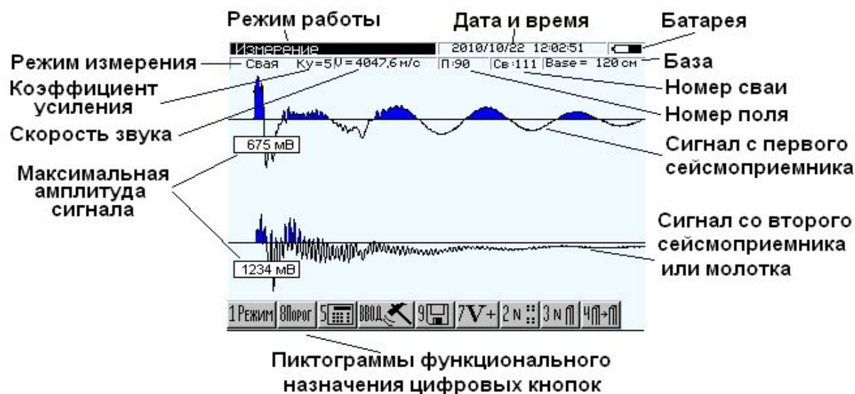
Рисунок 7 – Вид дисплея прибора в режиме измерений
