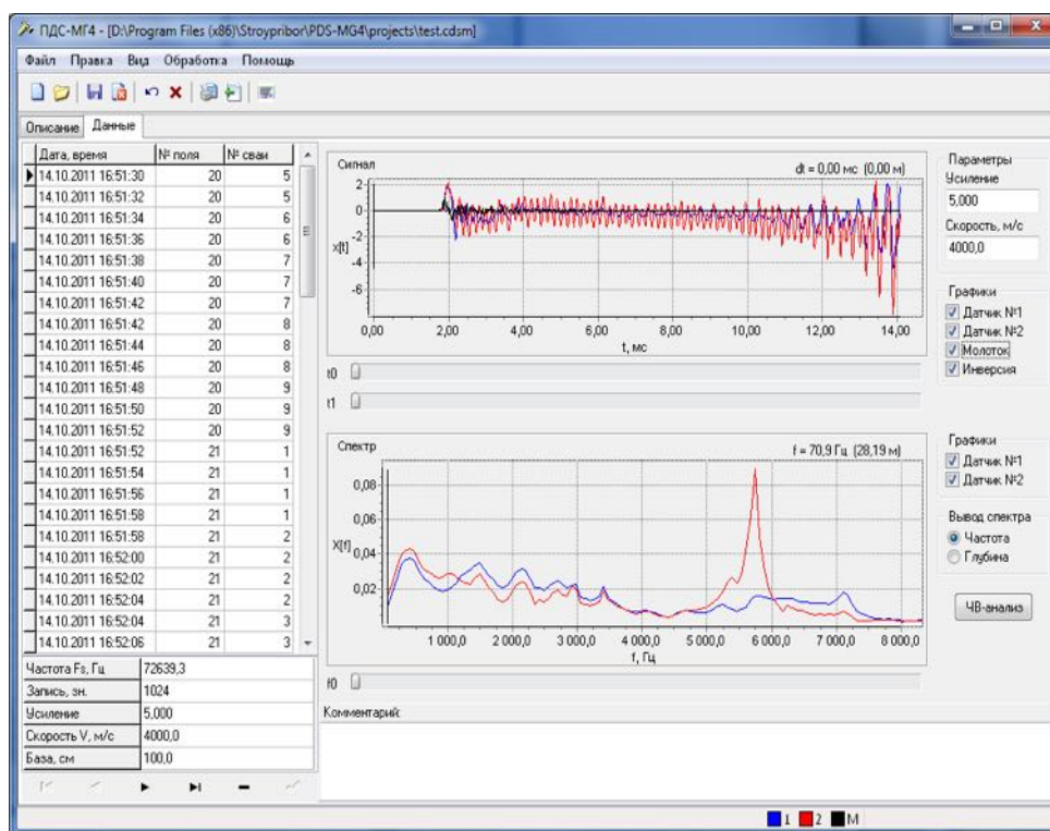
Рисунок 20 - Окно программы с прочитанными данными
